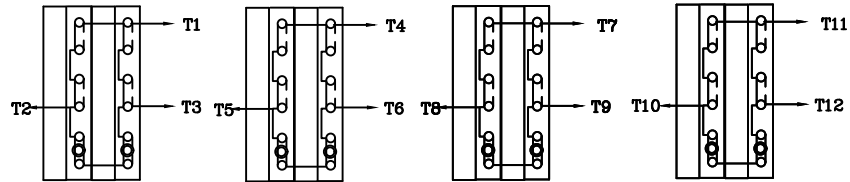
Bussing Diagram 460 Volt
